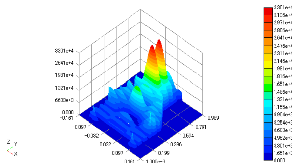
半導体処理装置中の電界分布
